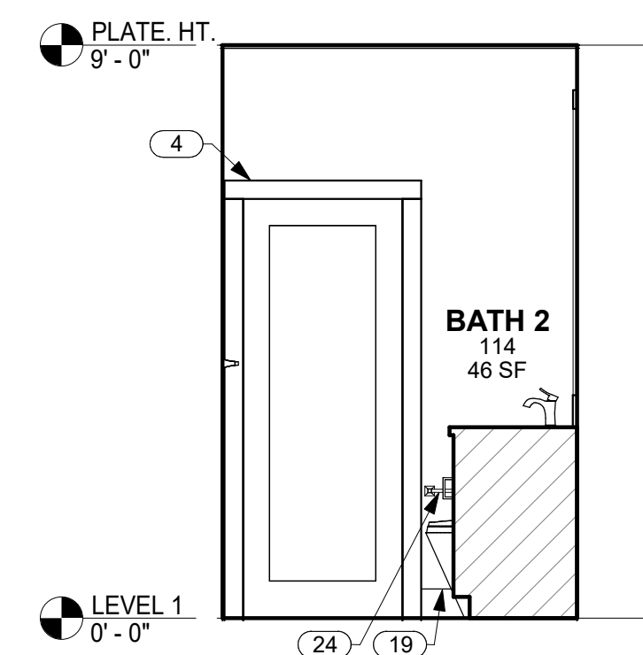
13 EAST WALL BATH 114 A7.0 SCALE: 3/8" = 1'-0"
