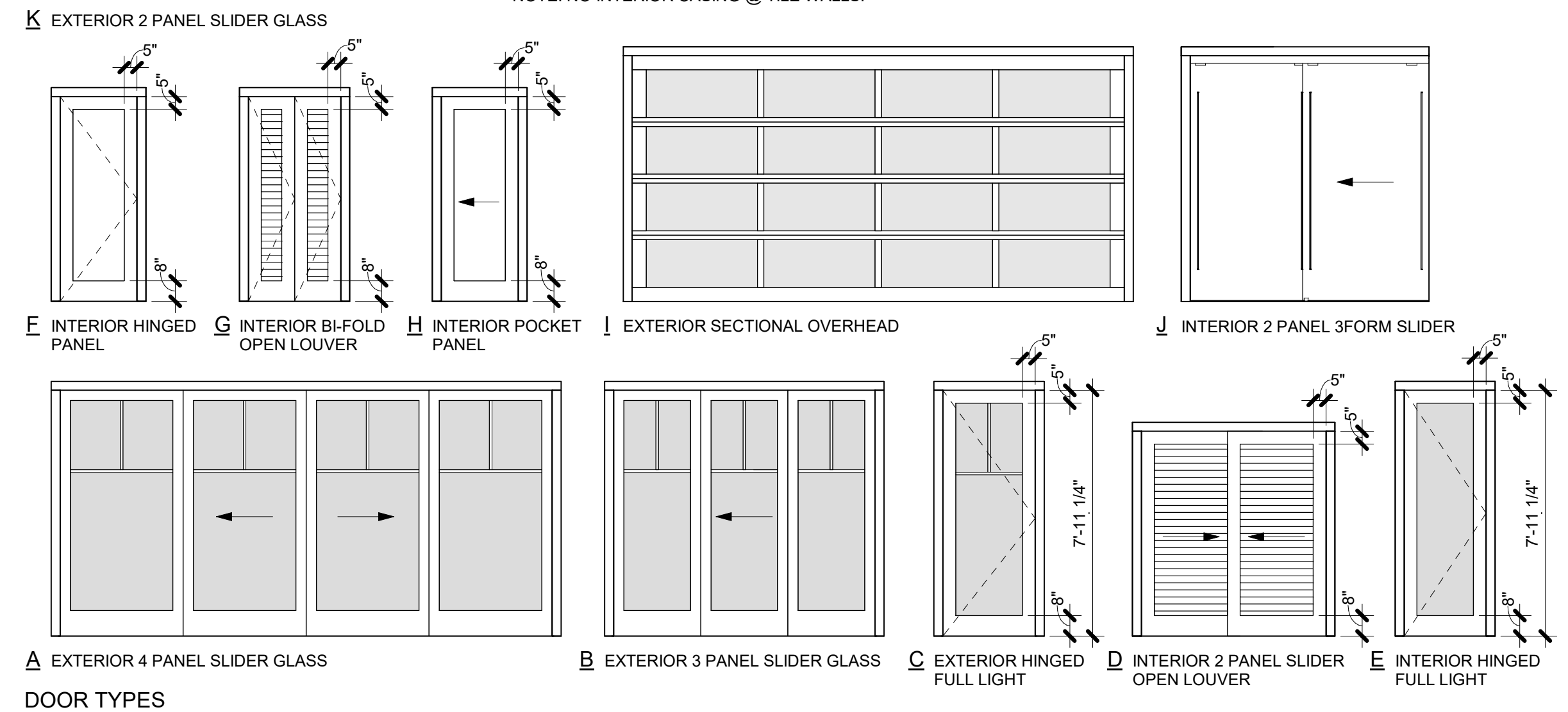
DOOR TYPES
