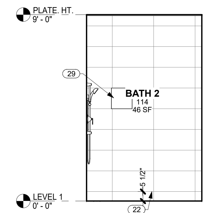
15 WEST WALL BATH 114 A7.0 SCALE: 3/8" = 1'-0"
