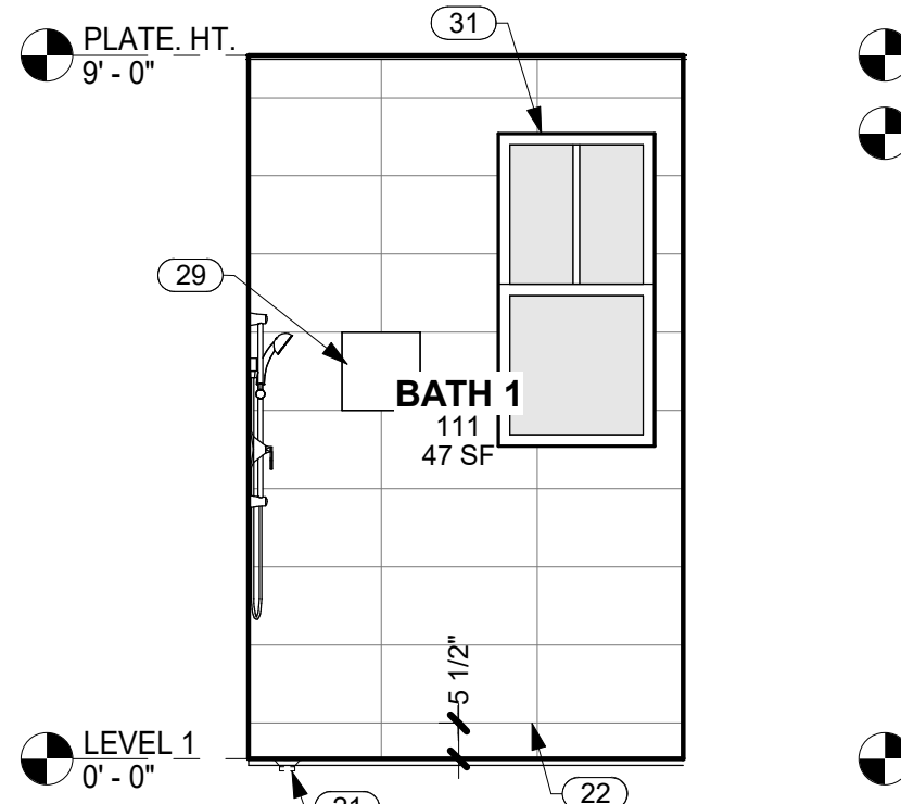
11 WEST WALL BATH 111 A7.0 SCALE: 3/8" = 1'-0"
