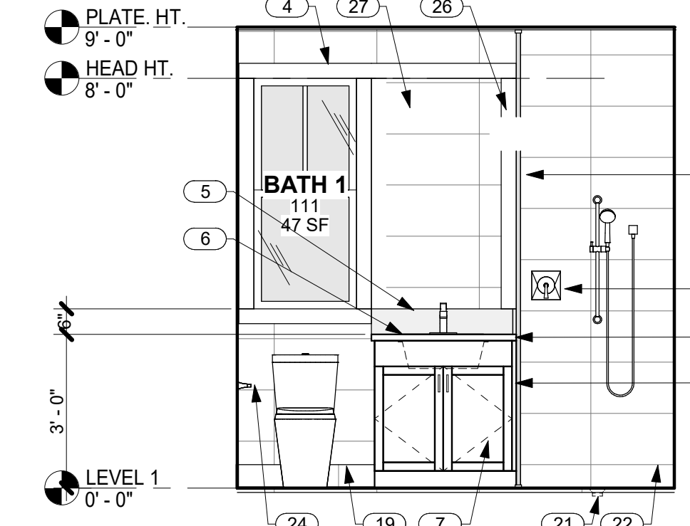
8 NORTH WALL BATH 111 A7.0 SCALE: 3/8" = 1'-0"
