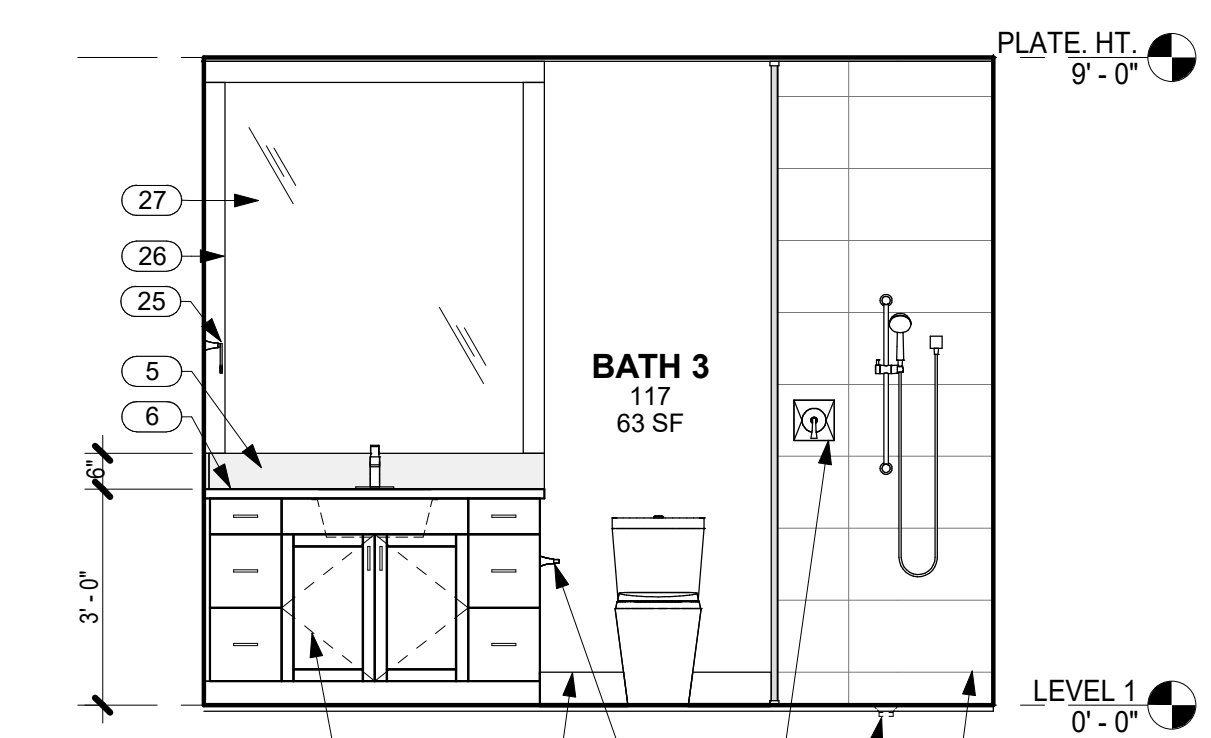
19 WEST WALL BATH 117 A7.0 SCALE: 3/8" = 1'-0"
