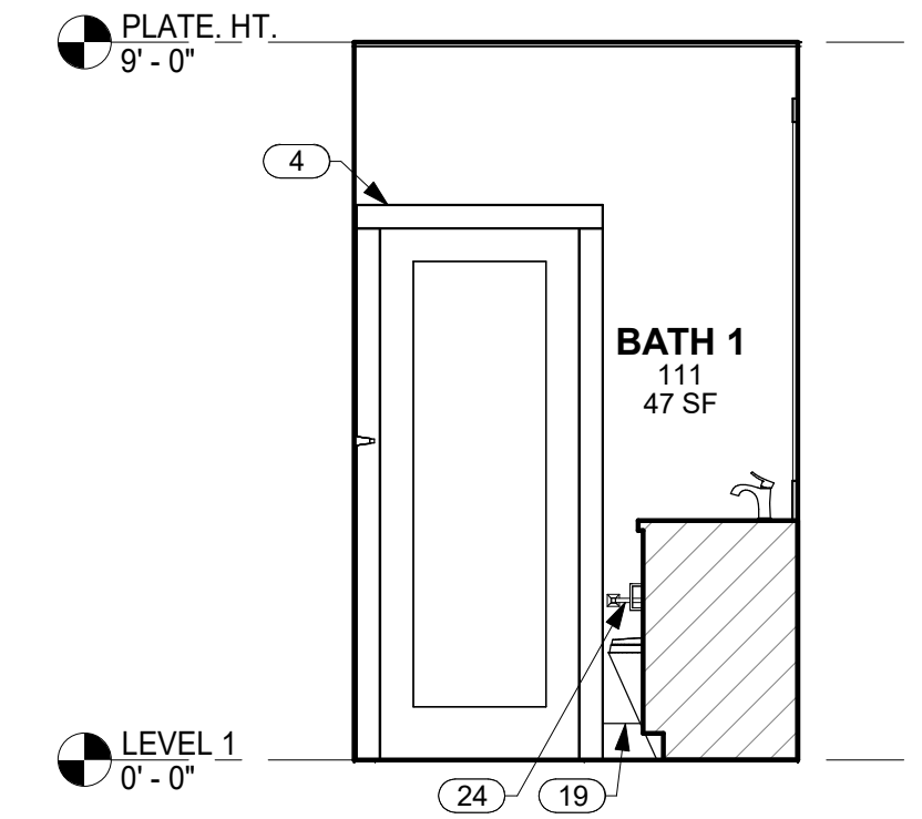
9 EAST WALL BATH 111 A7.0 SCALE: 3/8" = 1'-0"
