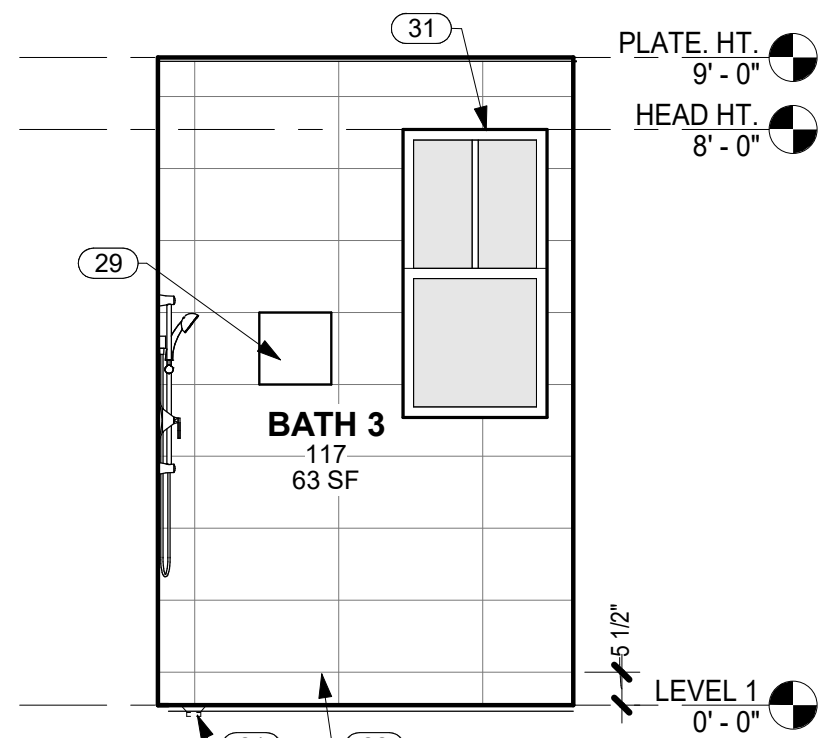
18 SOUTH WALL BATH 117 A7.0 SCALE: 3/8" = 1'-0"
