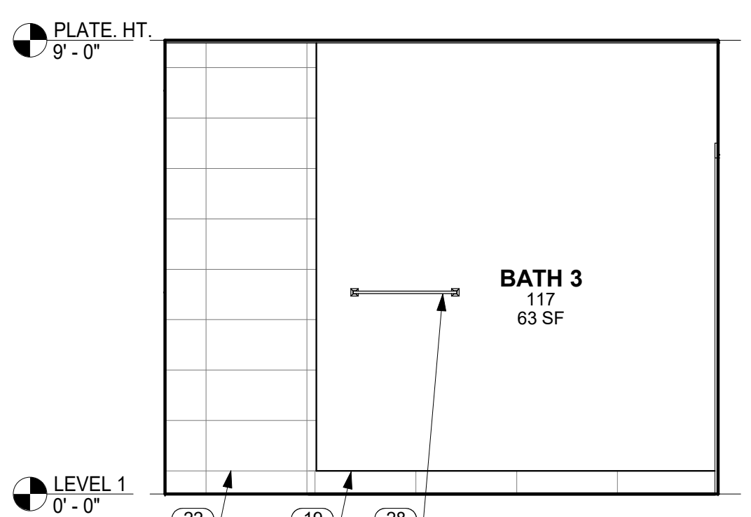
17 EAST WALL BATH 117 A7.0 SCALE: 3/8" = 1'-0"
