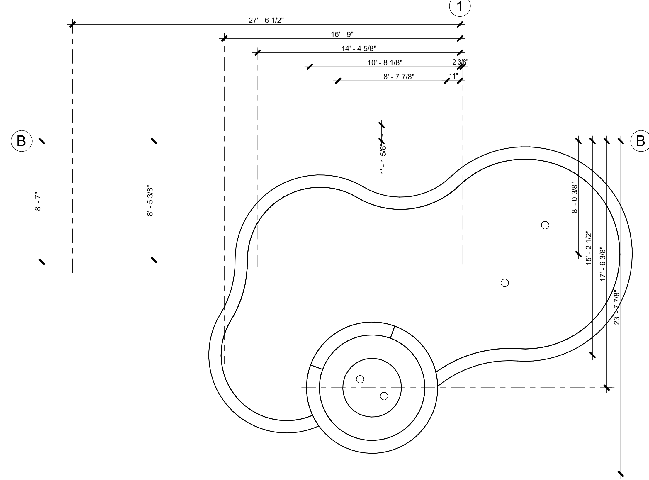
2 POOL LAYOUT A2.0 SCALE: 1/4" = 1'-0"
