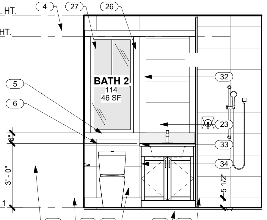
12 NORTH WALL BATH 114 A7.0 SCALE: 3/8" = 1'-0"
